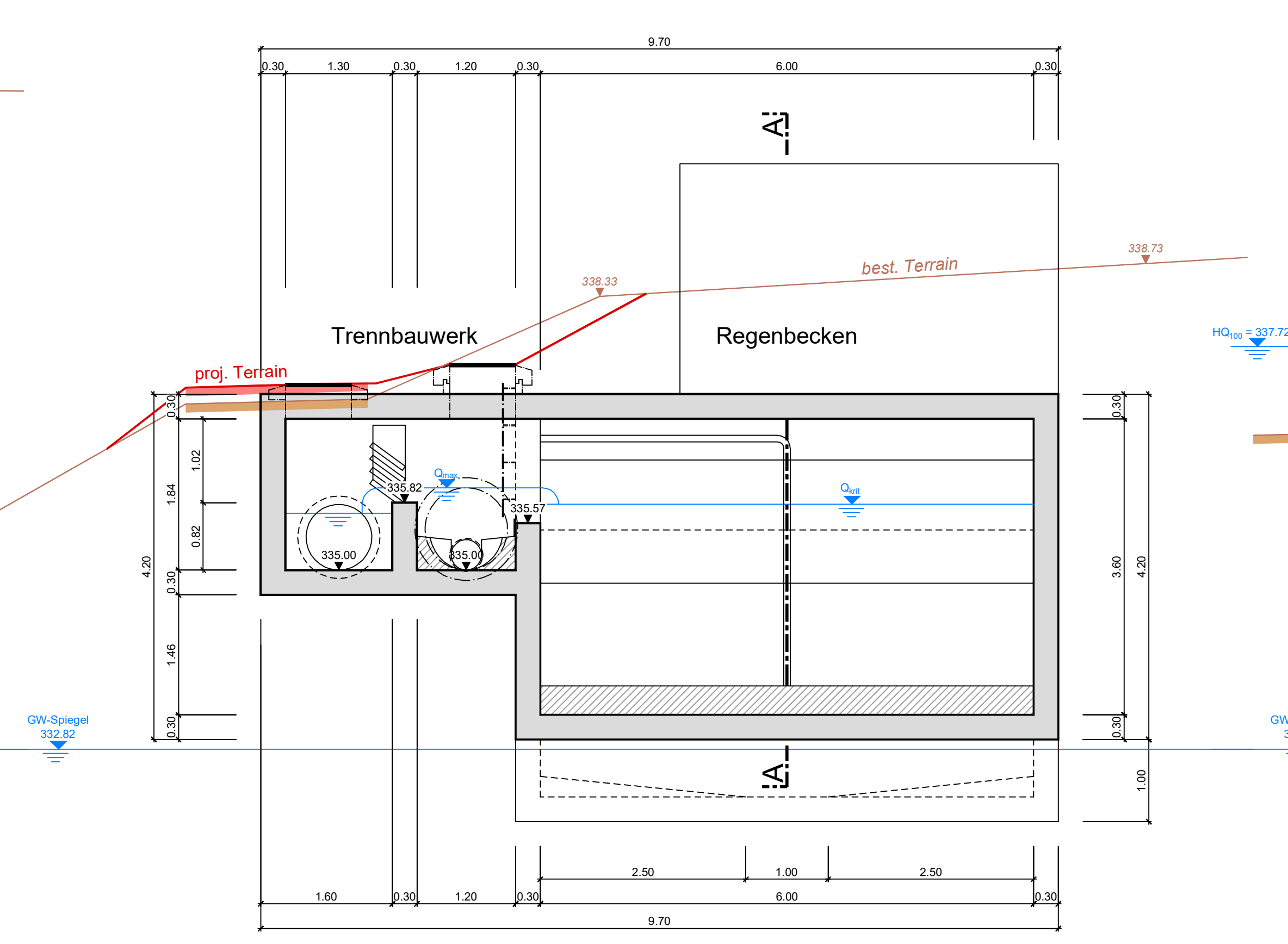
Schnitt B-B 1:50
