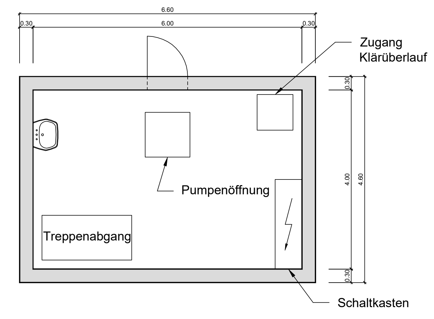
Grundriss Betriebsgebäude 1:50
