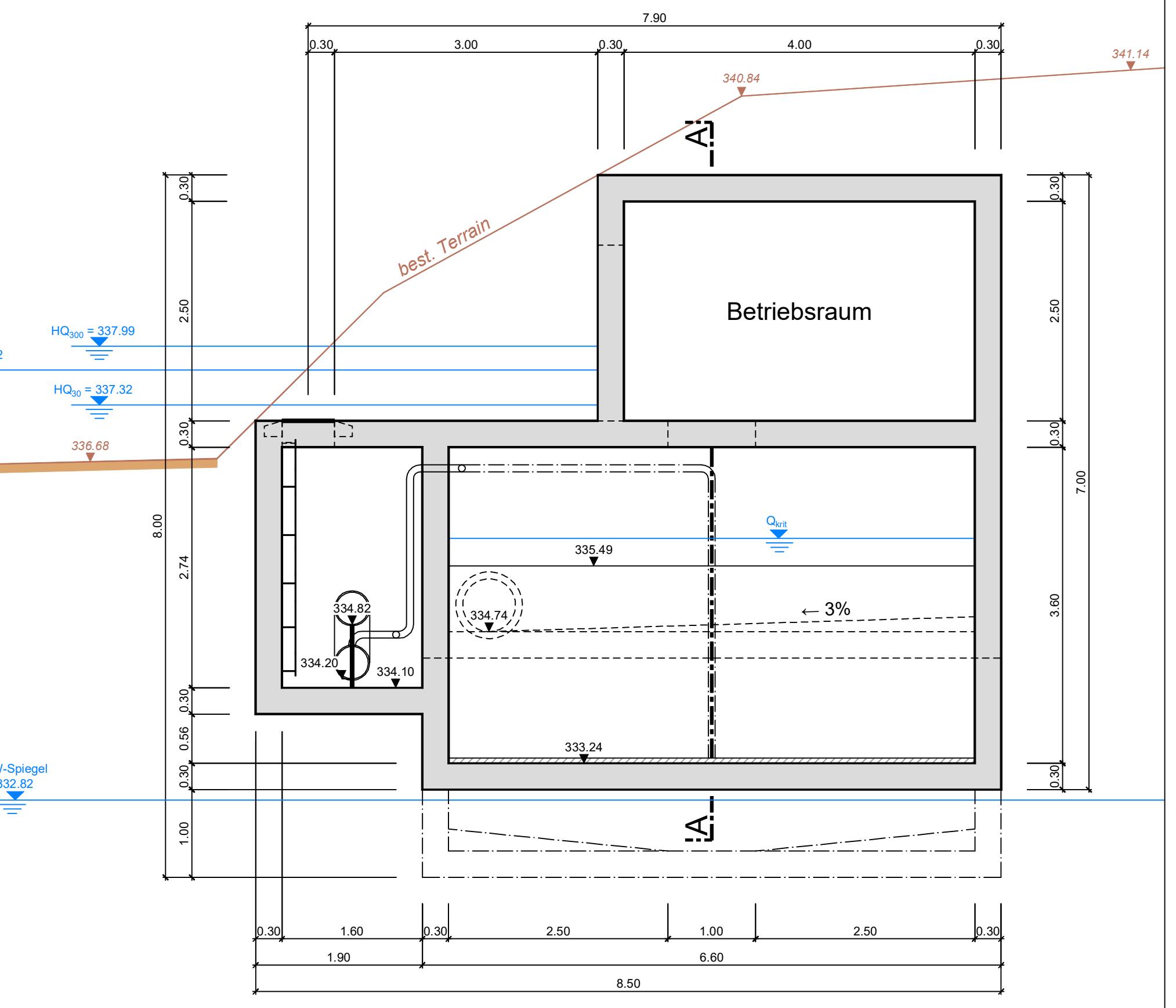
Schnitt C-C 1:50
